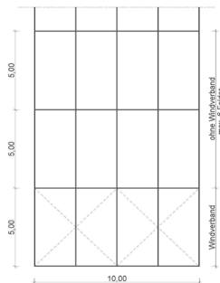
Draufsicht
